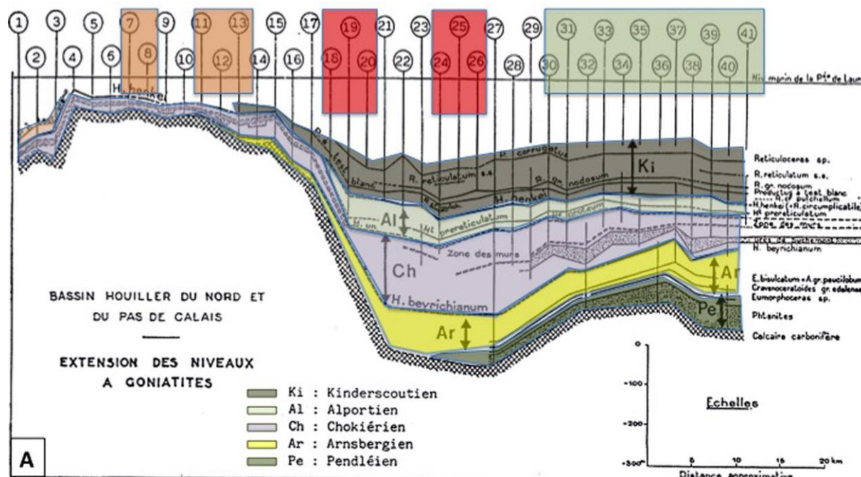
Article de Meilliez F. 2017, ASGNT24, fig. 8A : Carte et coupe ouest-est du bassin houiller du Nord et du Pas-de-Calais au Namurien. A – La coupe a été dessinée par Chalard (1960) en y reportant ses repères bio- et lithostratigraphiques identifiés en sondages. Meilliez (1989) a reporté (couleurs) les limites des sous-étages du Namurien (Paproth et al. , 1983). Les rectangles colorés regroupent des sondages qui participent à une même unité structurale. B – La carte localise tous les sondages analysés par Chalard (1960). Au moins trois unités structurales se distinguent par leur composition stratigraphique au Namurien. © SGN 2018.
